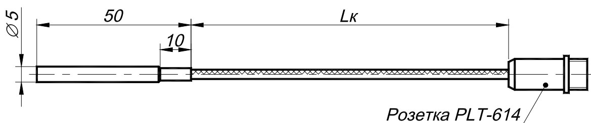
Габаритные размеры ПТСВ-2К-3
